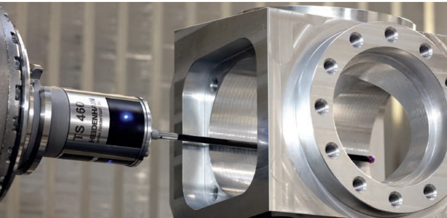
Kugeltaststift mit Kohlefaserschaft
