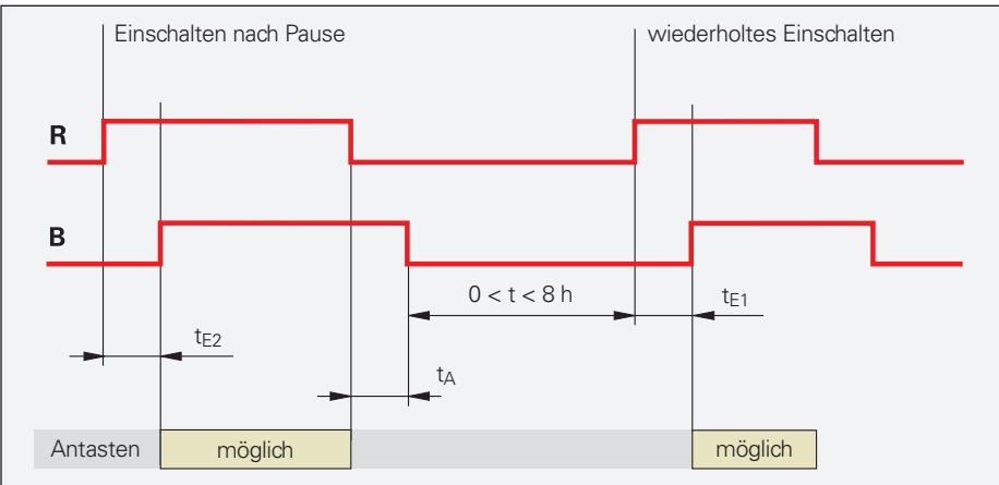
Ein- und Ausschalten des TS 460/TS 642/TS 760/TT 460
