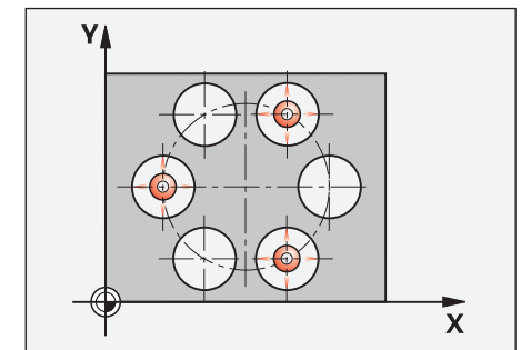
Lochkreis vermessen
