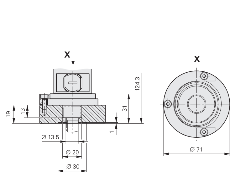
Montagesockel
