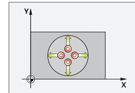
Kreistasche/Bohrung vermessen
