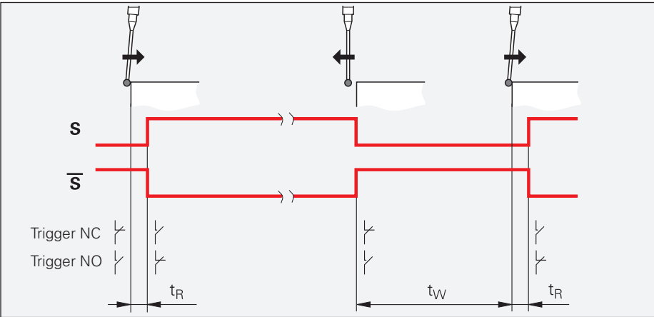
Schaltsignal bei TS 150/TS 750/TS 260/TT 160 Reaktionszeit t_R \leq 10 \mu\text{s} Wiederholabstand t_W > 25 \text{ ms}
